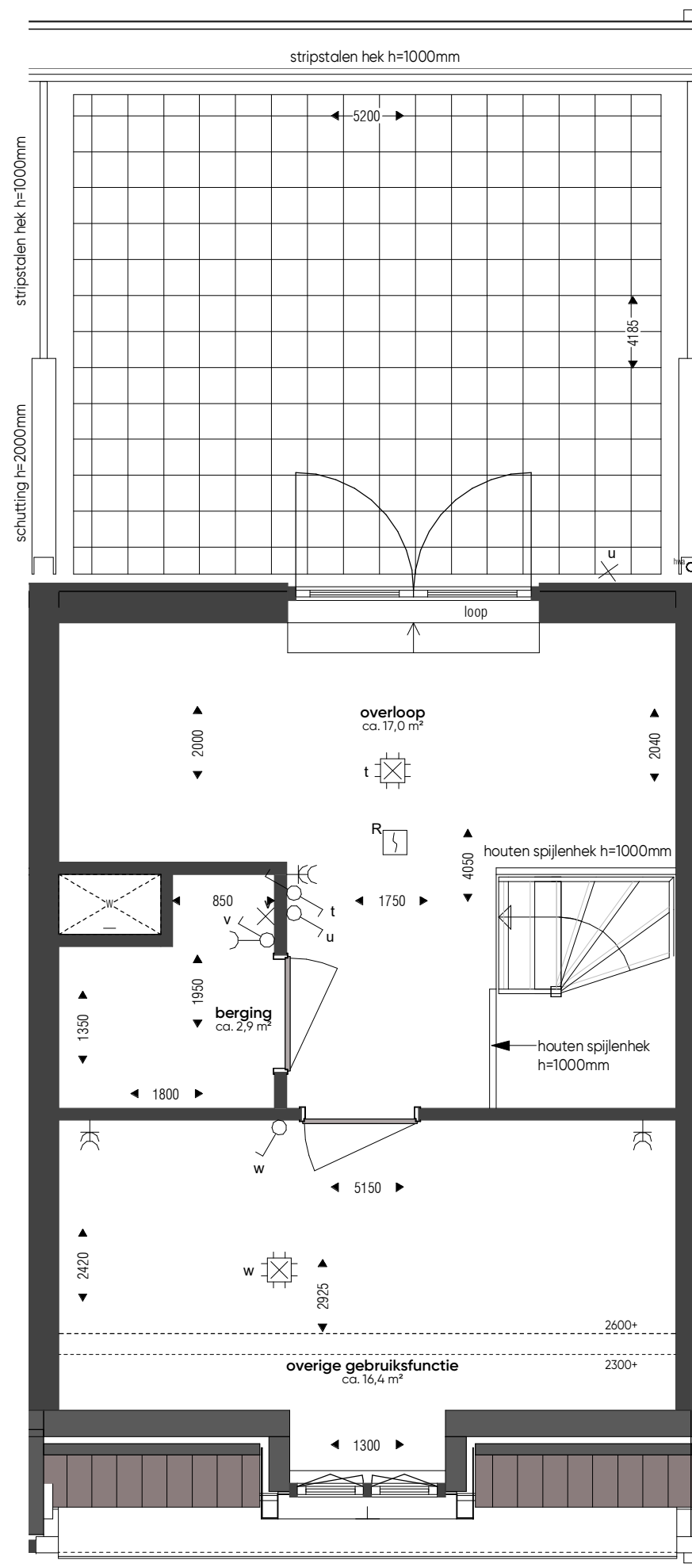
3e verdieping_wtype C-39_bnr. 120 schaal: 1:50
