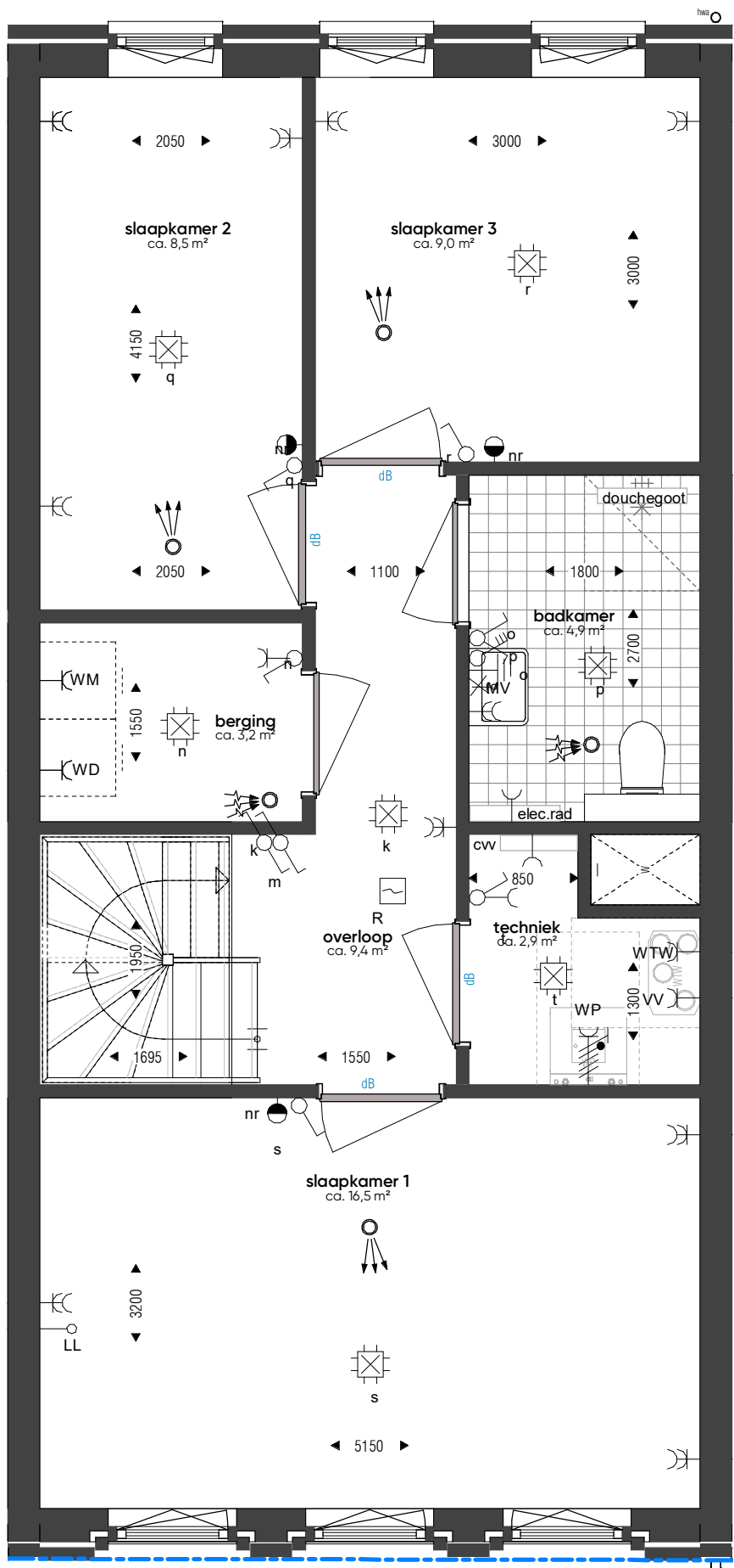
2e verdieping_wtype B-35_bnr. 111
