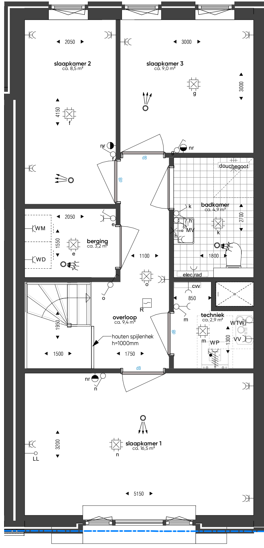
2e verdieping_wtype B-34_bnr. 107
