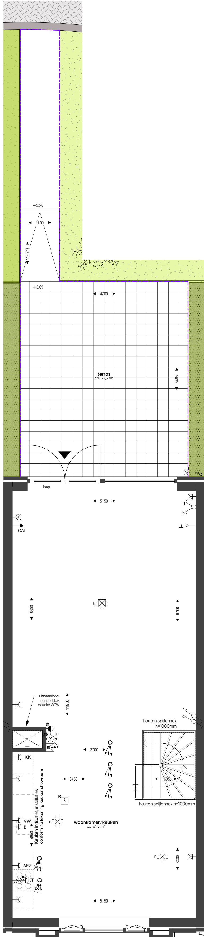
1e verdieping_wtype C-39_bnr. 120 schaal: 1:50
