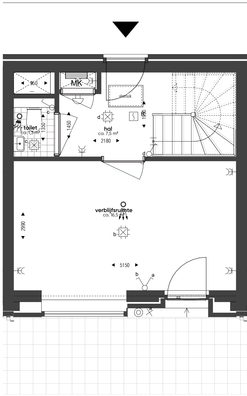
begane grond_wtype C-39_bnr. 121 schaal: 1:50
