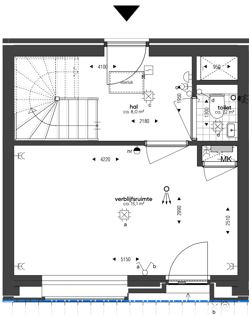
begane grond_wtype B-34_bnr. 109
