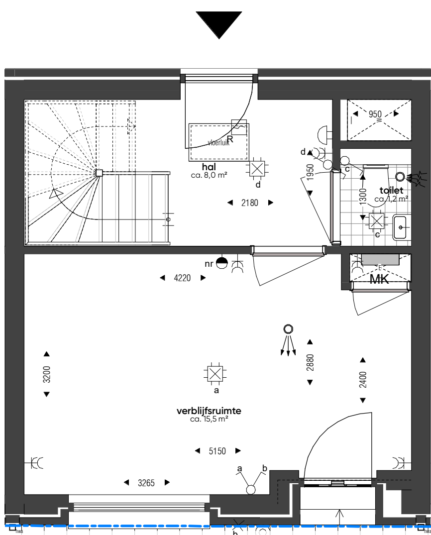
begane grond_wtype B-36_bnr. 113
