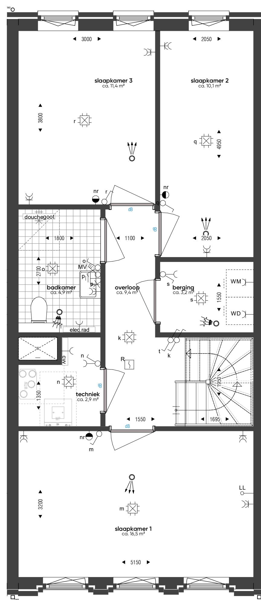
2e verdieping_wtype C-40_bnr. 123 schaal: 1:50
