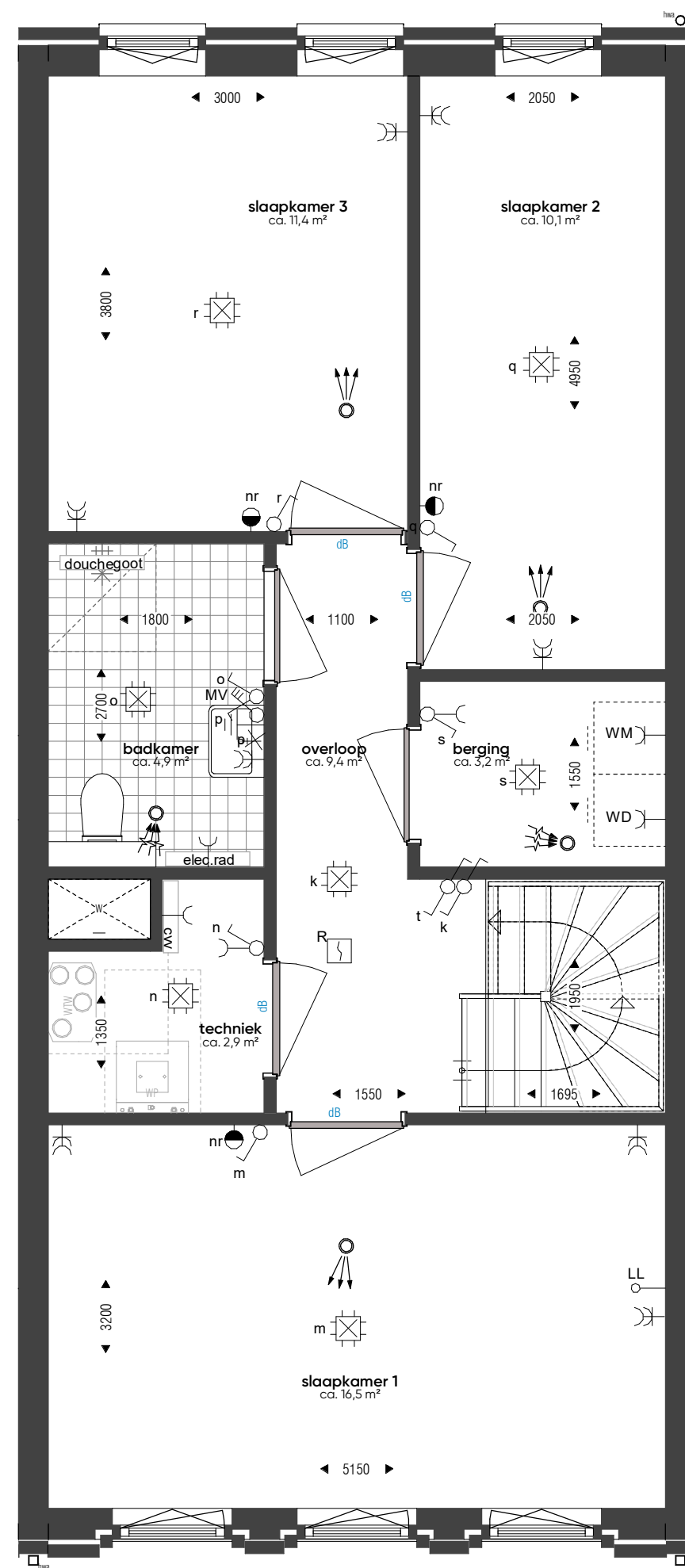
2e verdieping_wtype C-40_bnr. 122 schaal: 1:50
