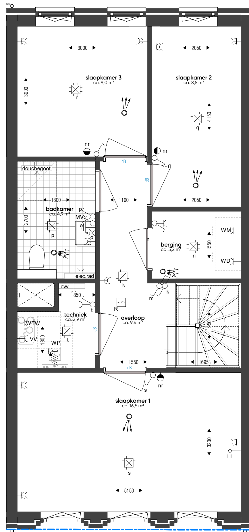
2e verdieping_wtype B-35_bnr. 112
