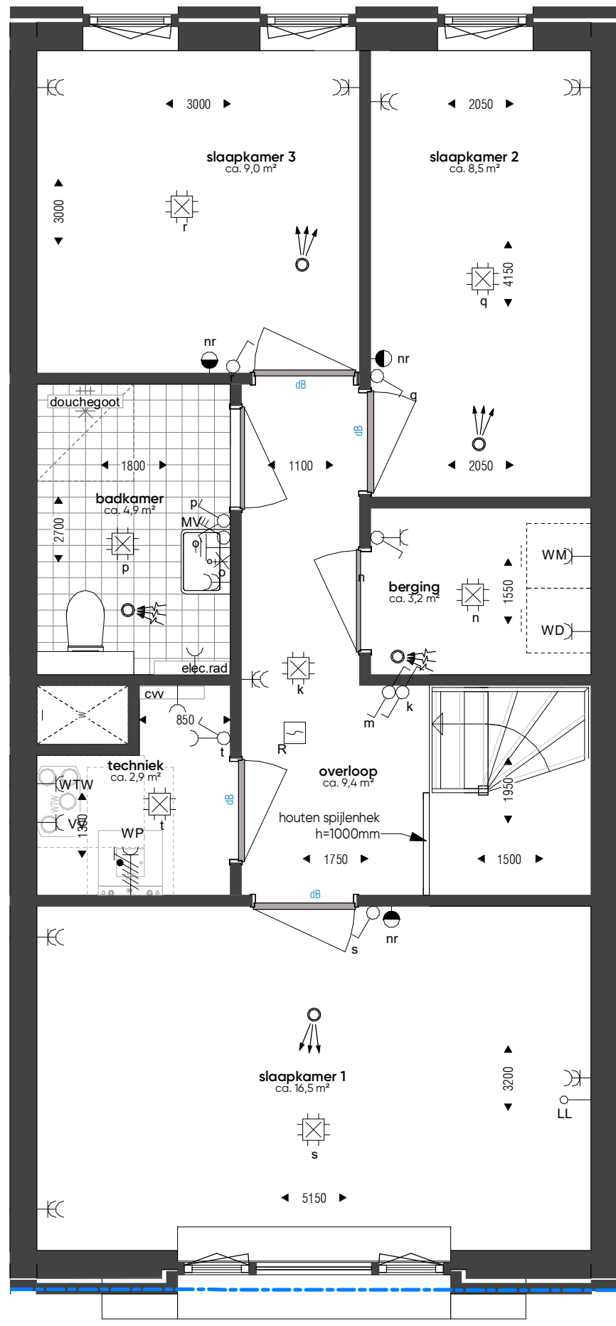
2e verdieping_wtype B-34_bnr. 108
