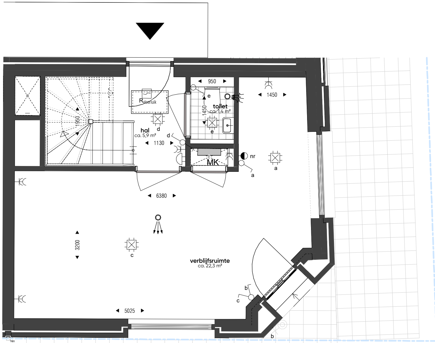
begane grond_wtype B-37_bnr. 115
