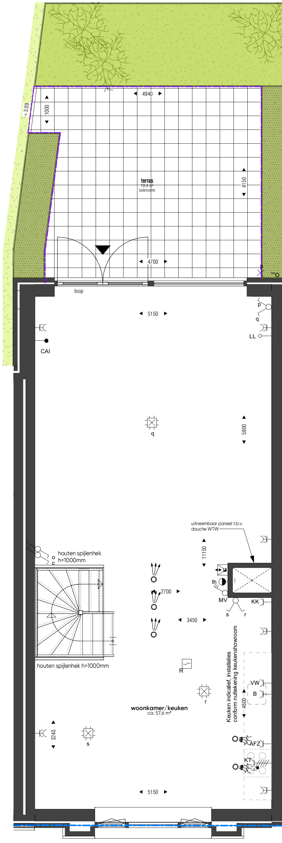
1e verdieping_wtype B-34_bnr. 107
