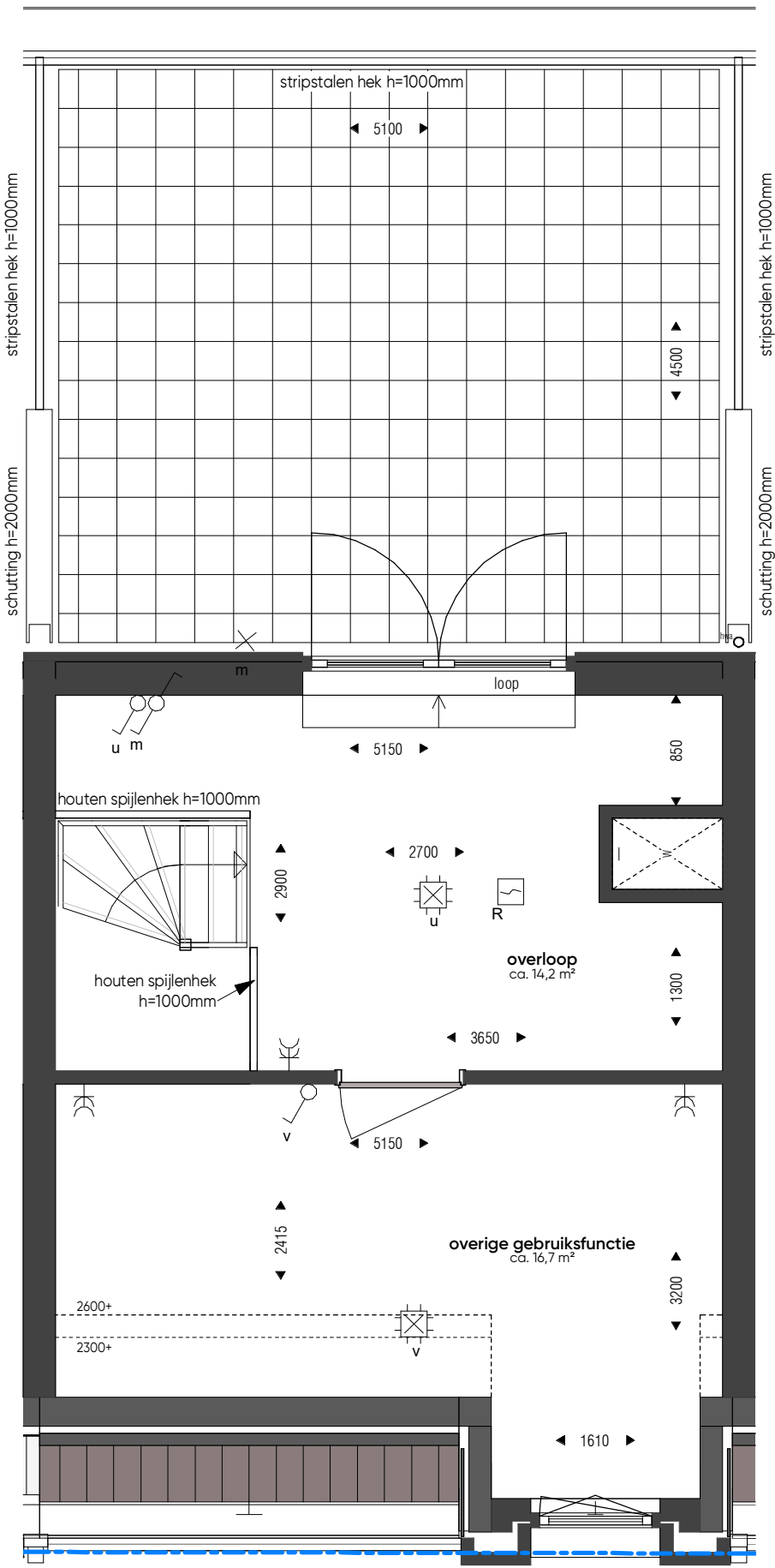
3e verdieping_wtype B-36_bnr. 113
