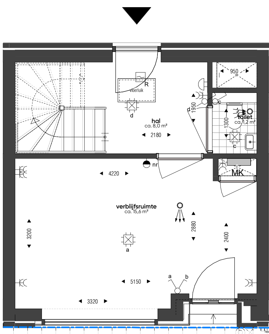
begane grond_wtype B-35_bnr. 111
