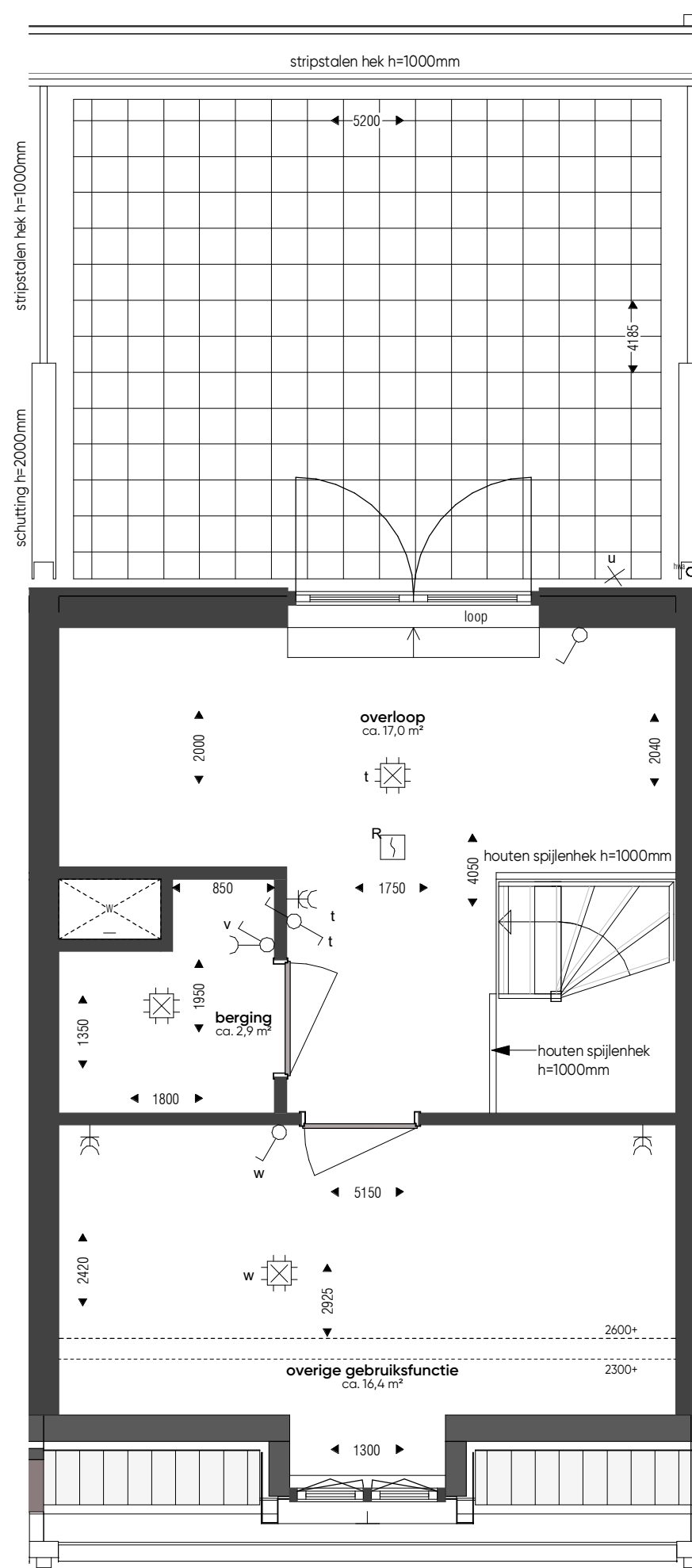
3e verdieping_wtype C-40_bnr. 122 schaal: 1:50
