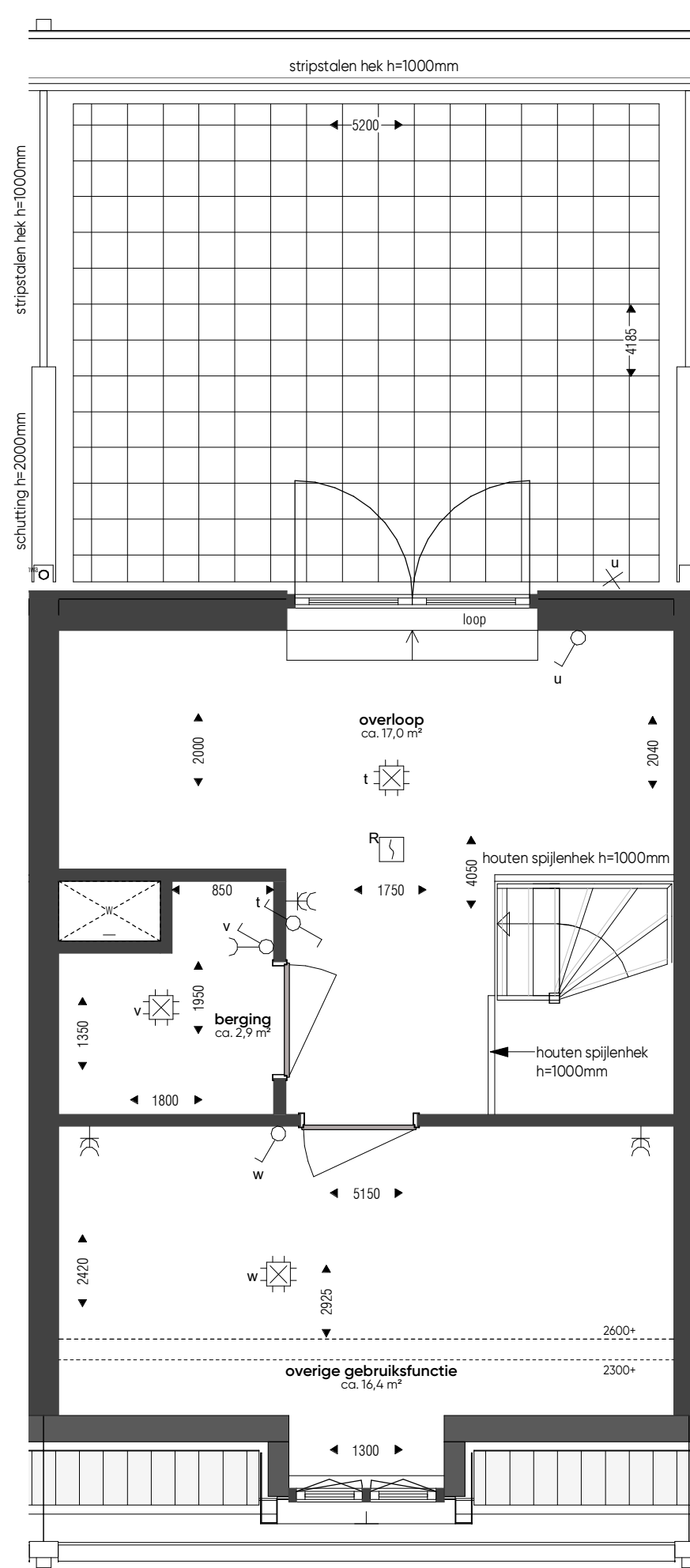
3e verdieping_wtype C-40_bnr. 123 schaal: 1:50
