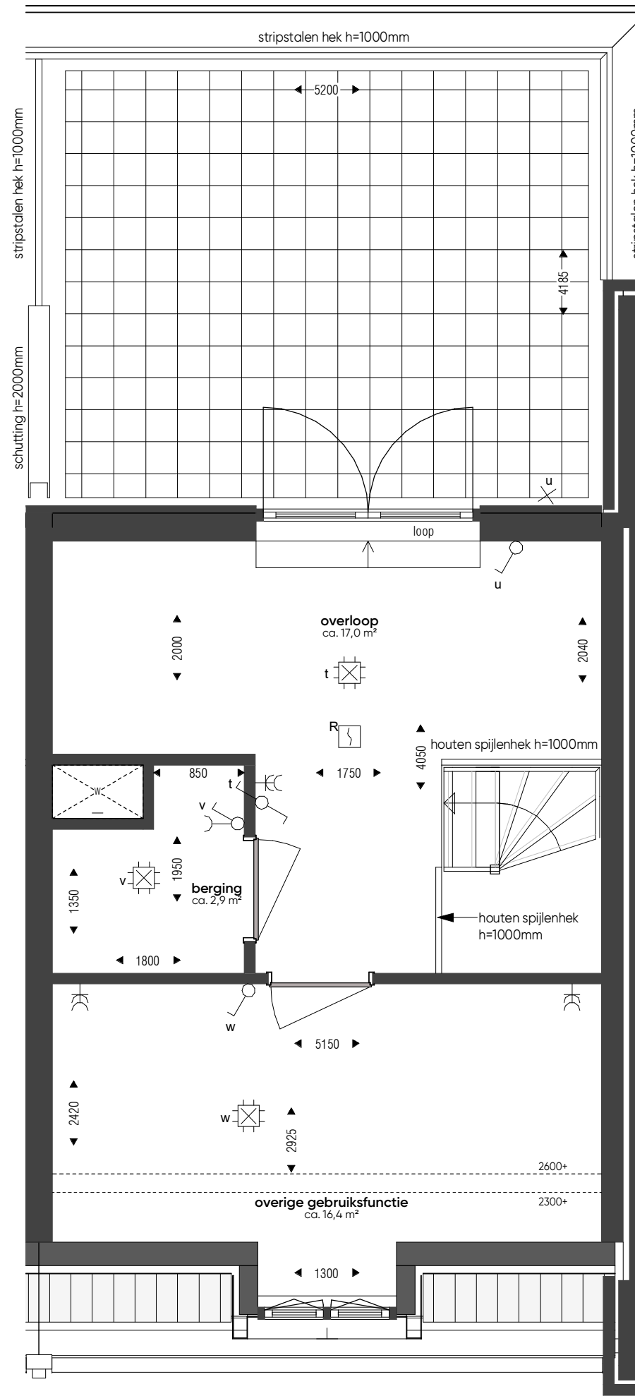
3e verdieping_wtype C-40_bnr. 124 schaal: 1:50
