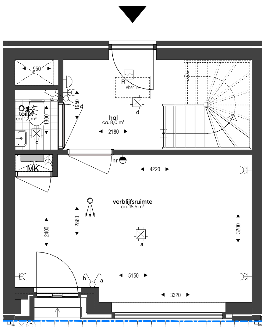
begane grond_wtype B-35_bnr. 112
