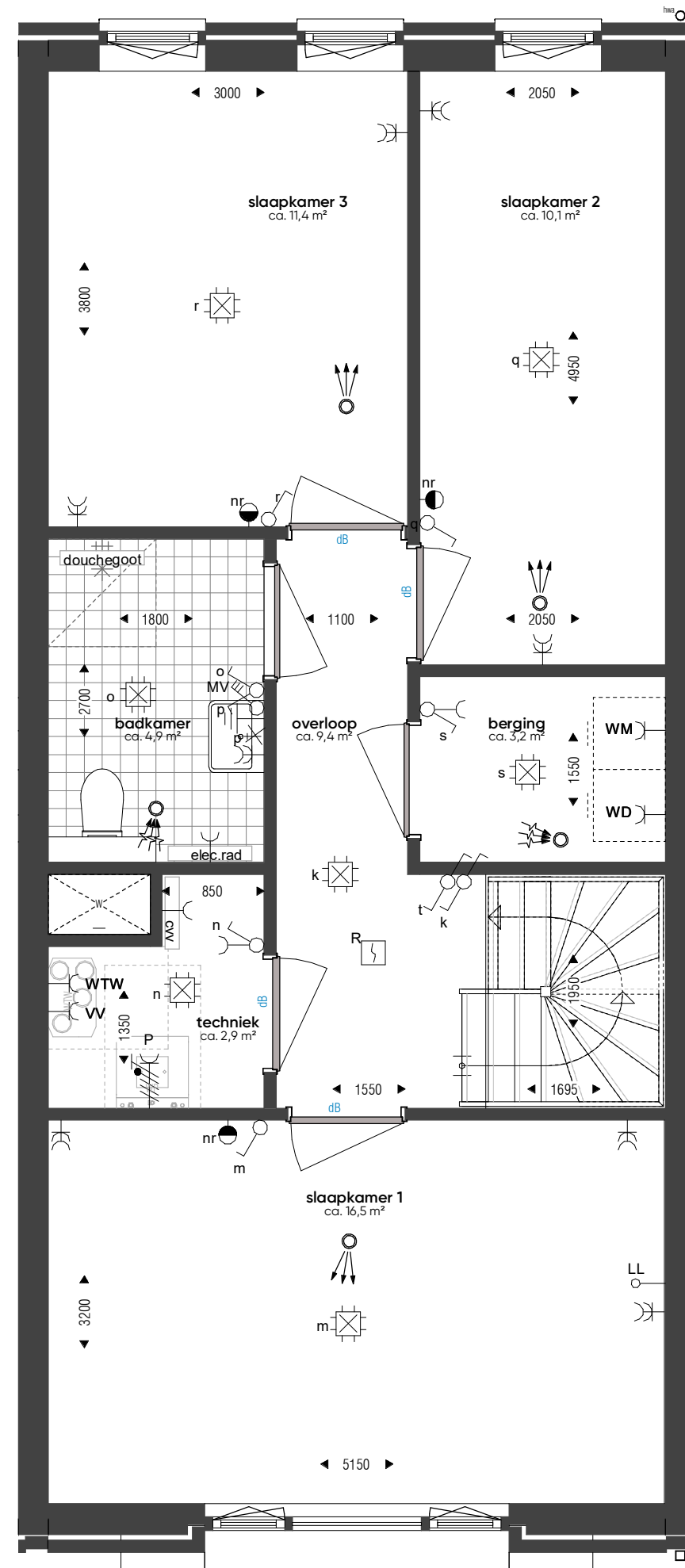
2e verdieping_wtype C-39_bnr. 120 schaal: 1:50
