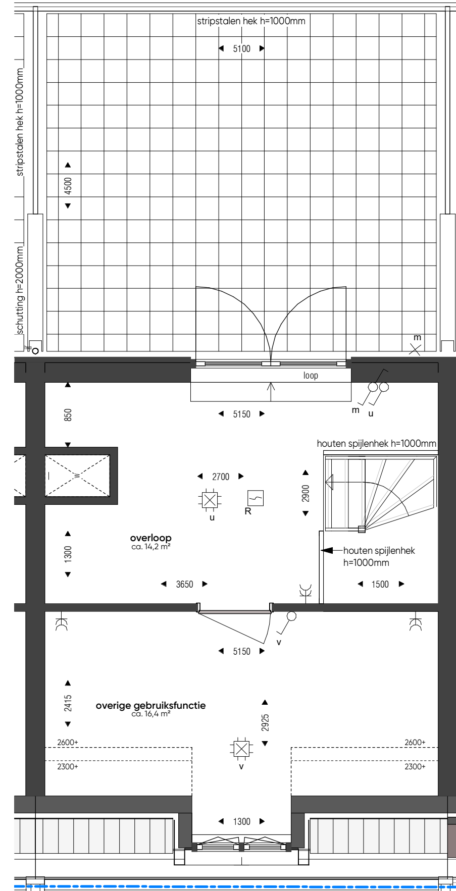
3e verdieping_wtype B-35_bnr. 112
