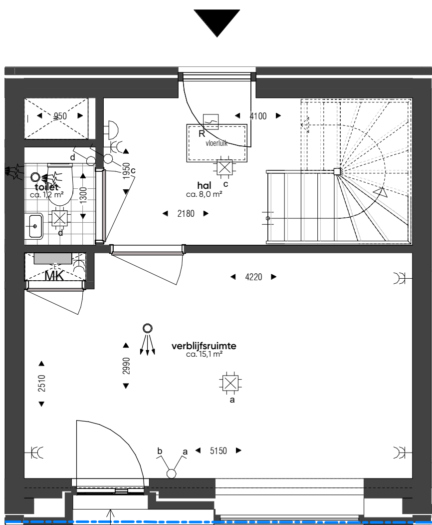
begane grond_wtype B-34_bnr. 108
