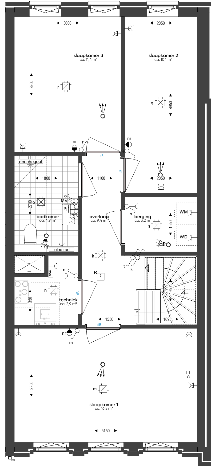
2e verdieping_wtype C-40_bnr. 124 schaal: 1:50
