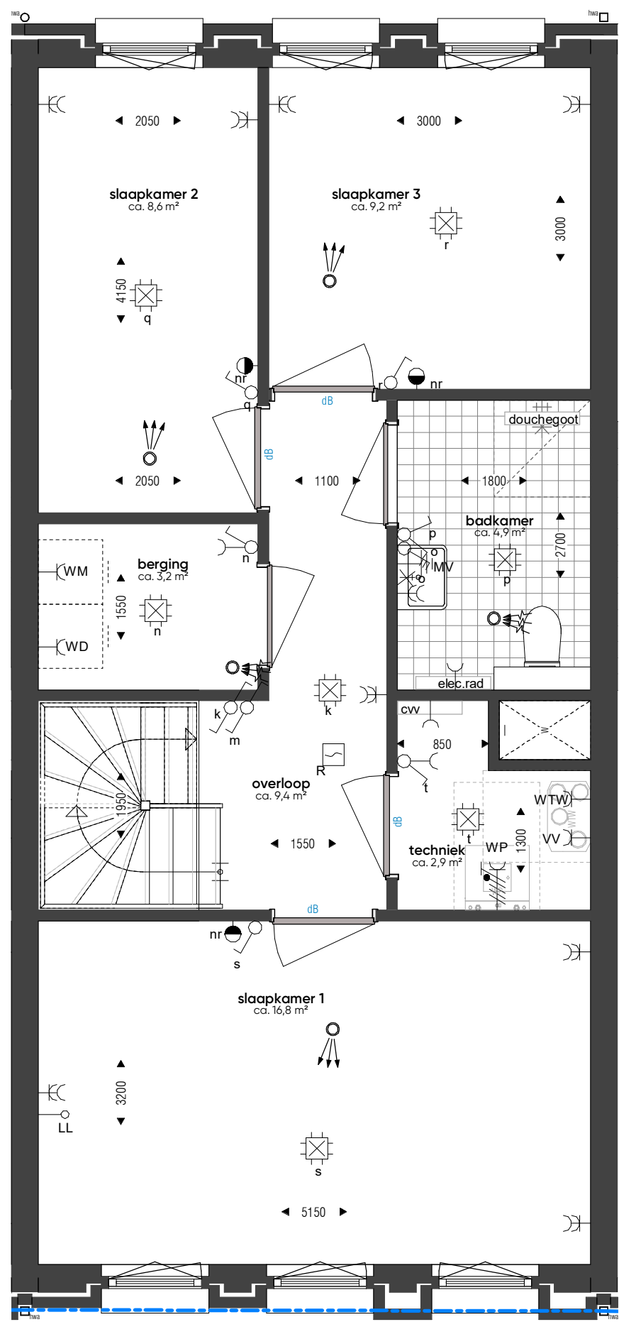
2e verdieping_wtype B-36_bnr. 114
