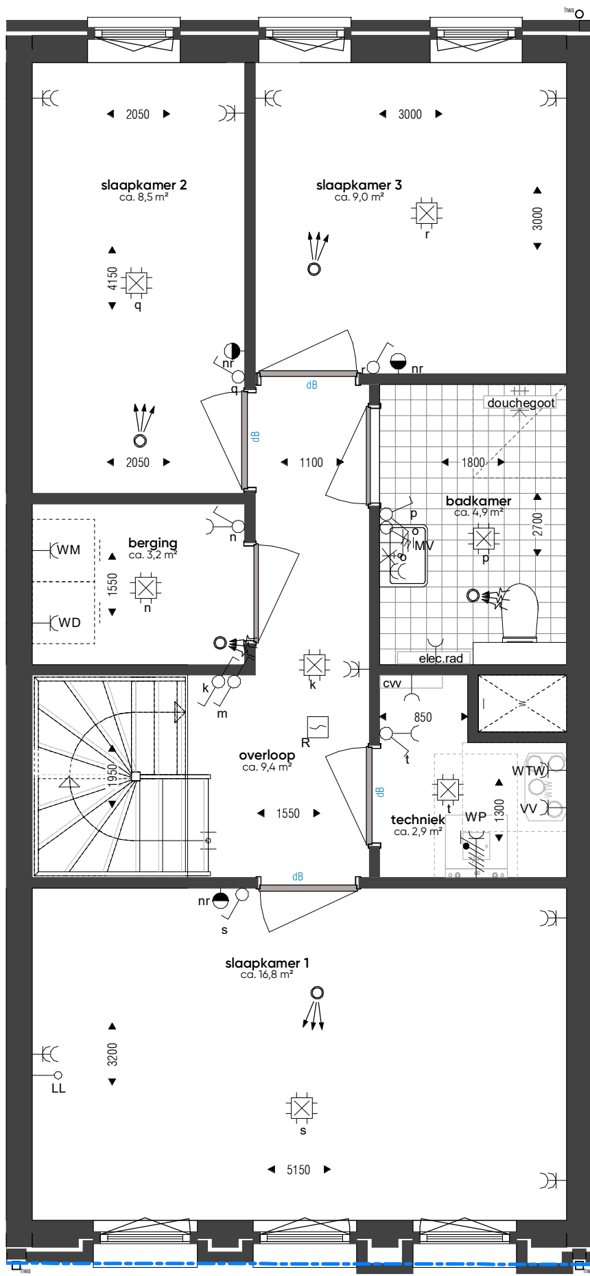
2e verdieping_wtype B-36_bnr. 113
