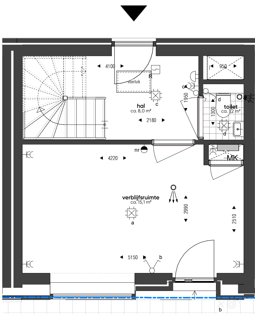
begane grond_wtype B-34_bnr. 107
