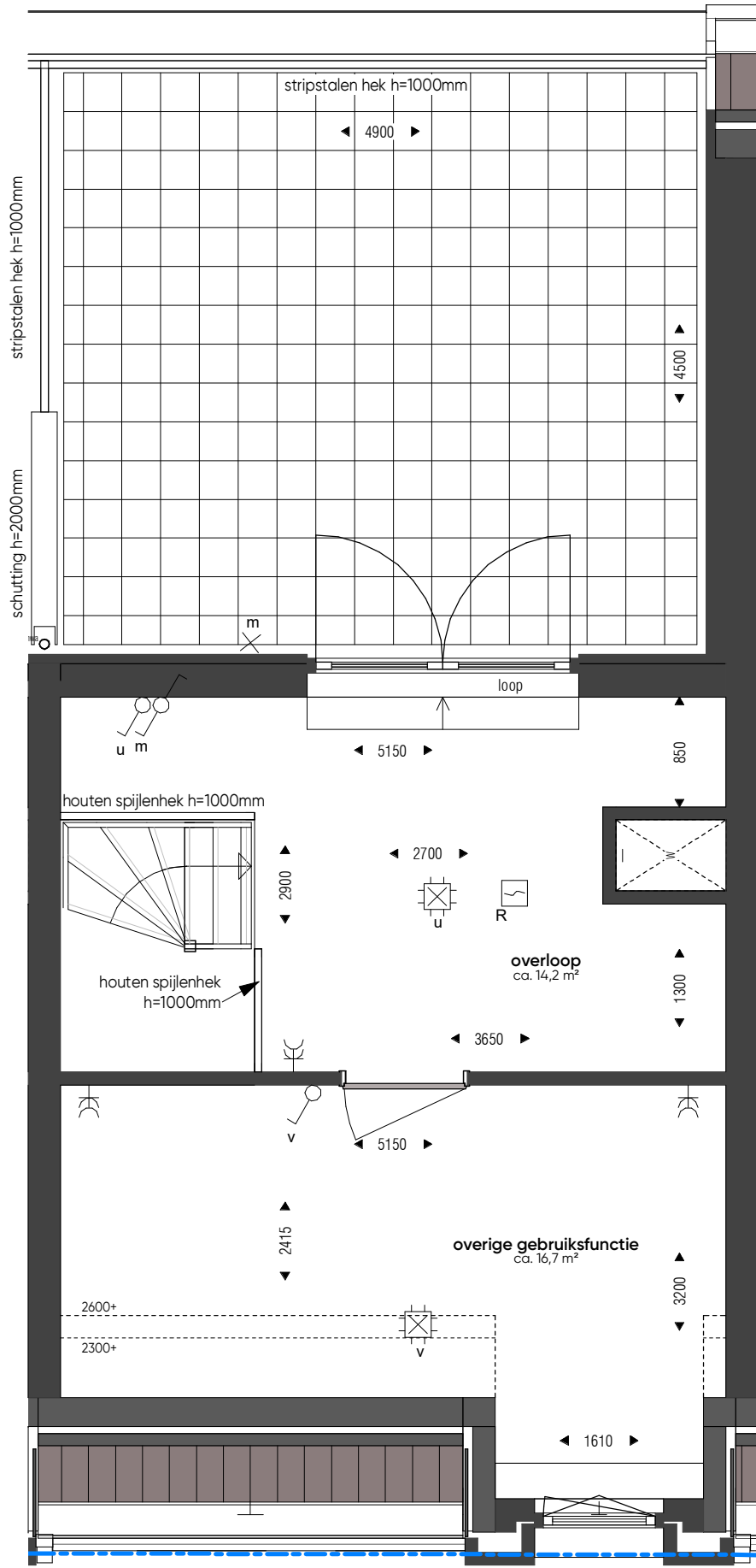
3e verdieping_wtype B-36_bnr. 114
