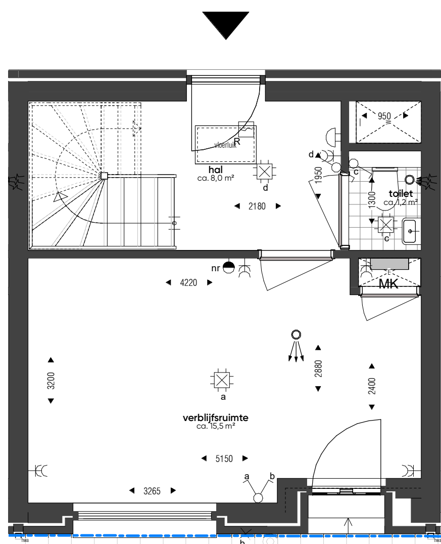
begane grond_wtype B-36_bnr. 114
