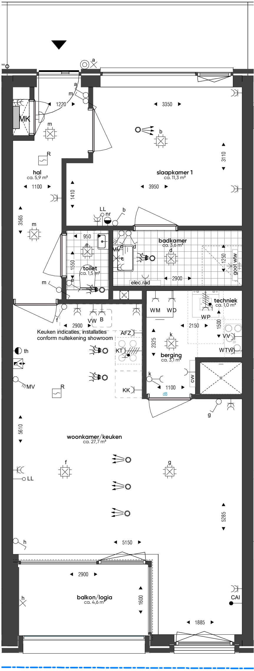
2e verdieping_wtype D-48_bnr. 136 schaal: 1 : 50
