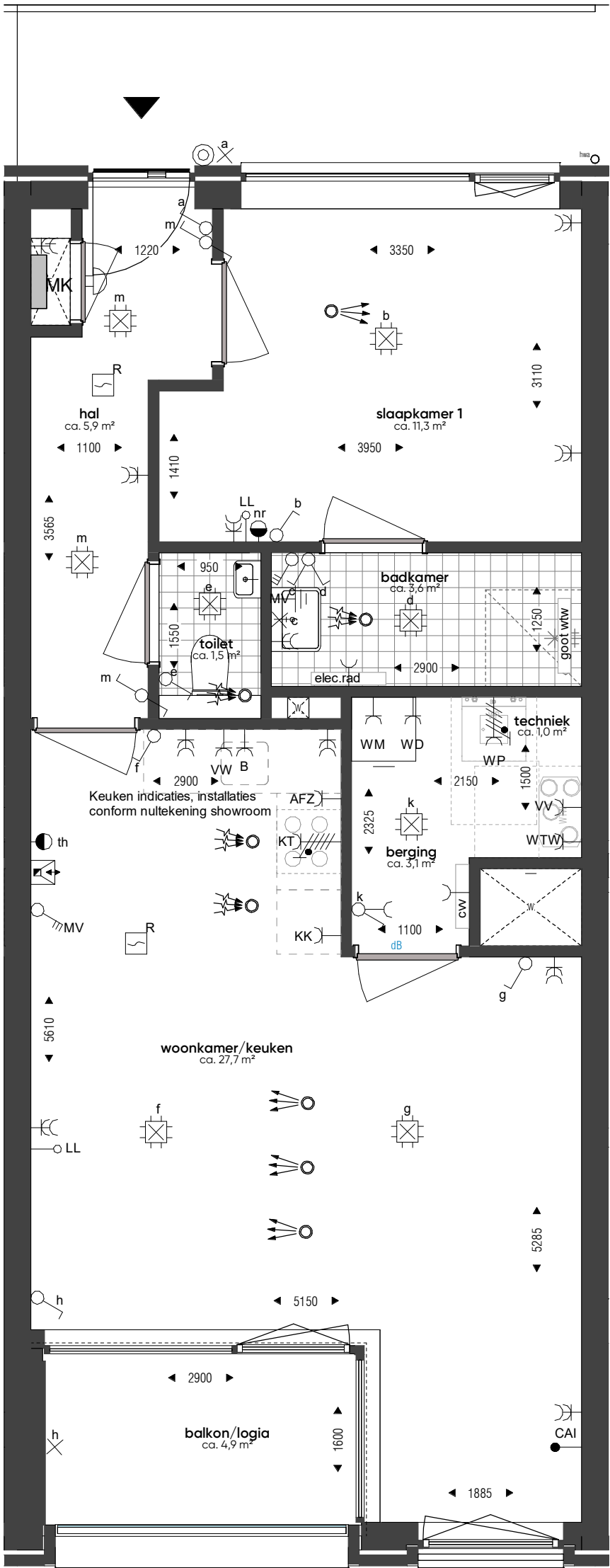
3e verdieping_wtype D-47_bnr. 143 schaal: 1 : 50
