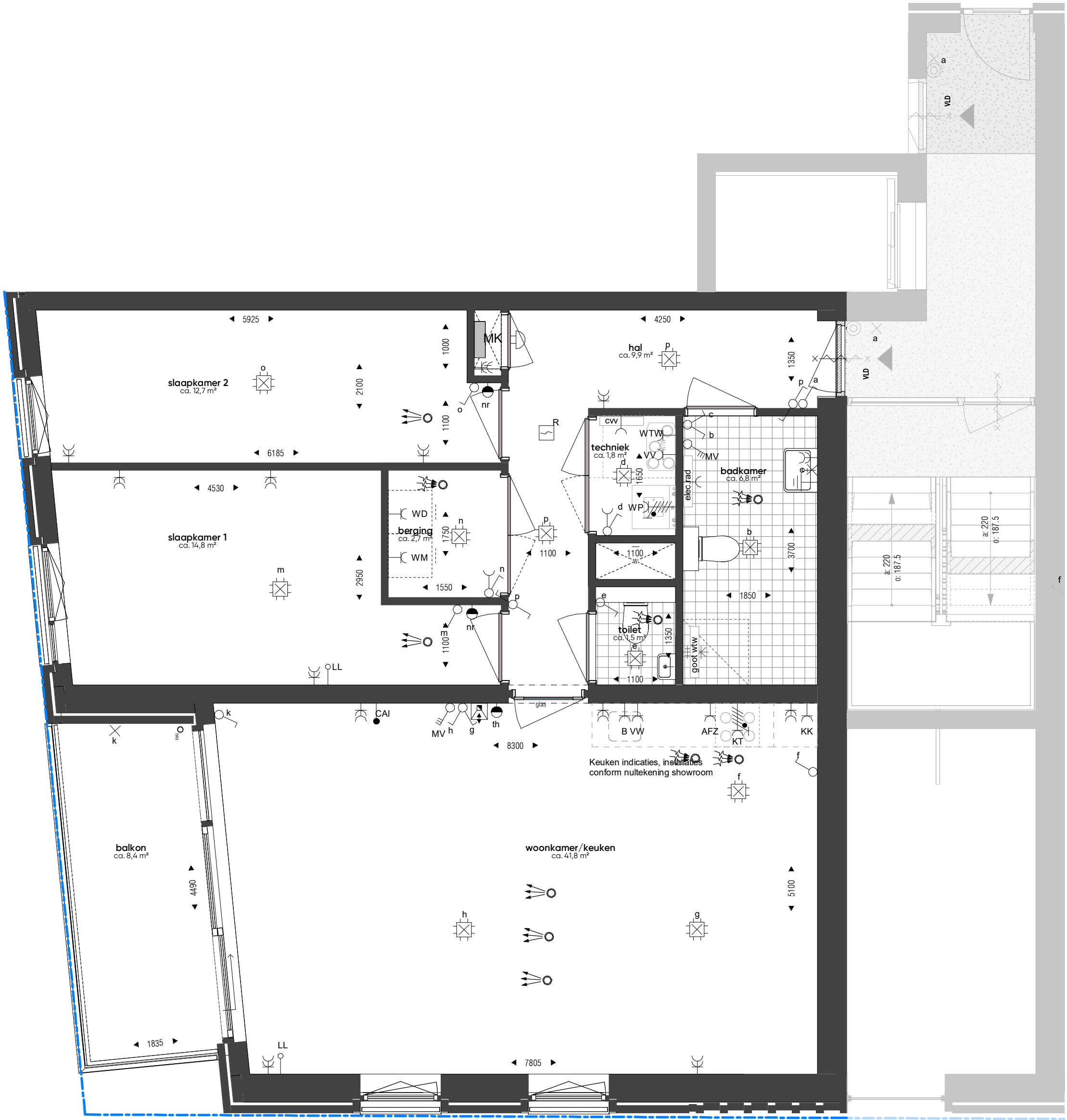
1e verdieping_wtype D-46_bnr. 132 schaal: 1 : 50
