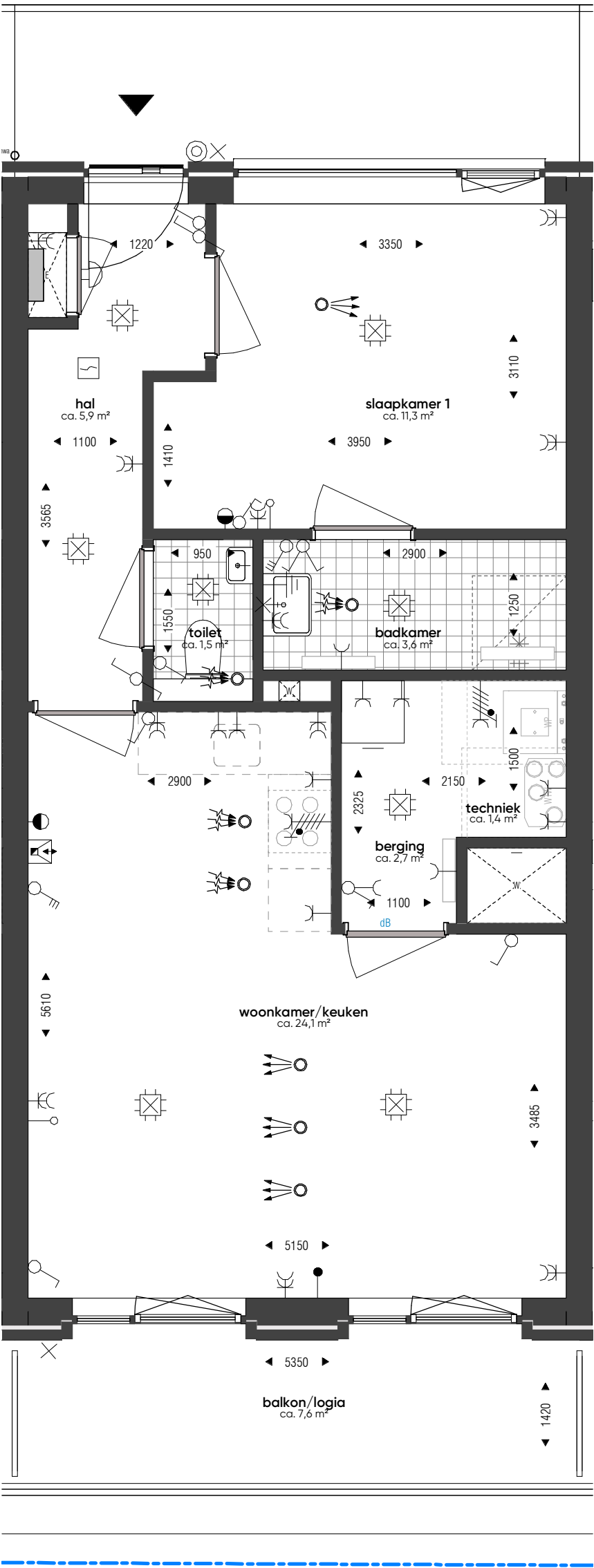
4e verdieping_wtype D-50_bnr. 148 schaal: 1 : 50
