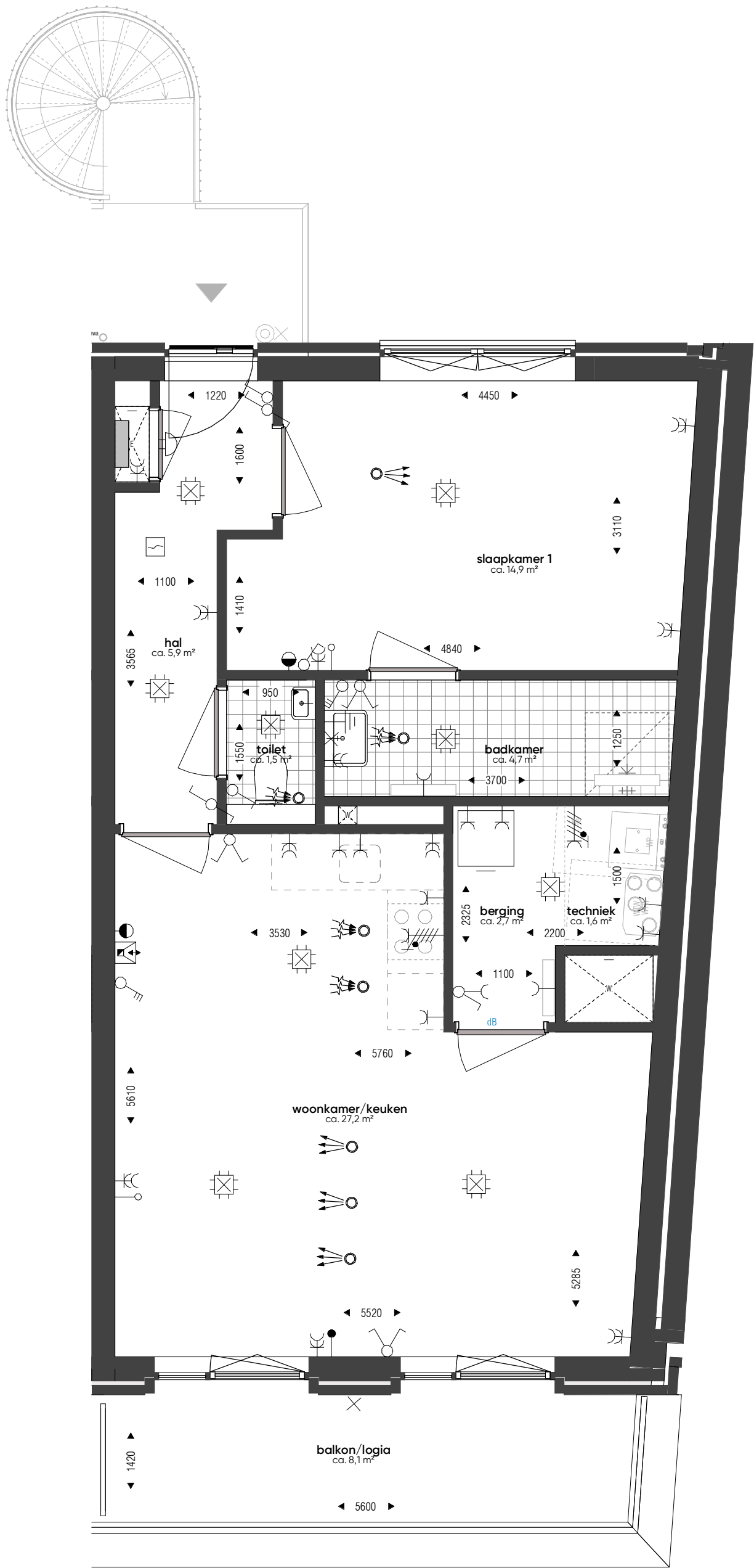
4e verdieping_wtype D-51_bnr. 150
