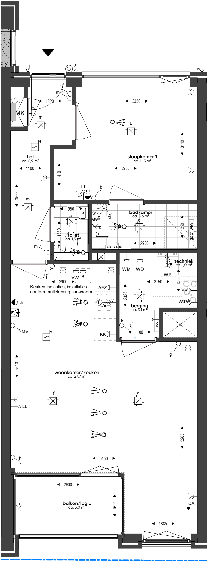
3e verdieping_wtype D-47_bnr. 141
