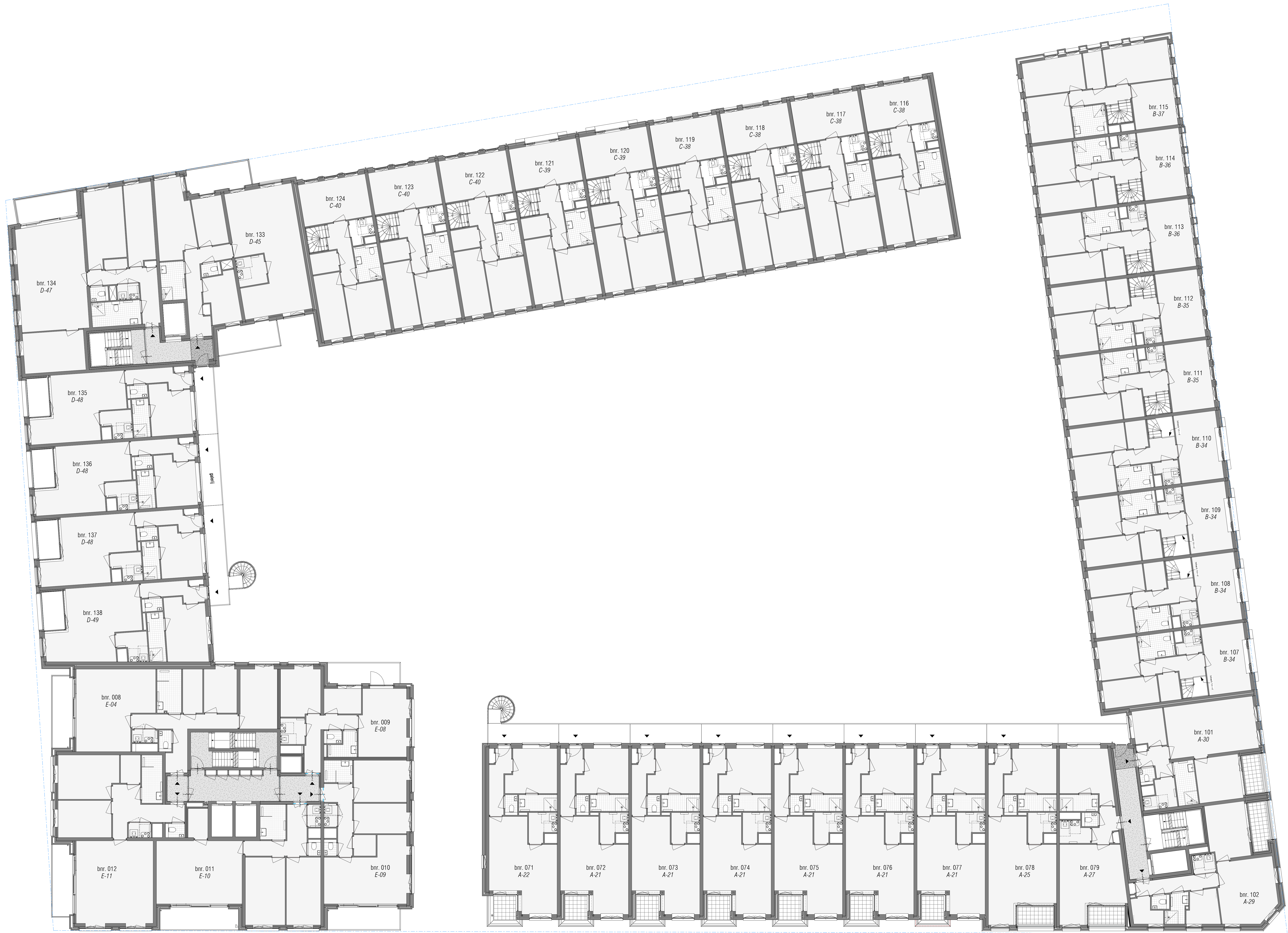
2e verdieping schaal: 1:100
