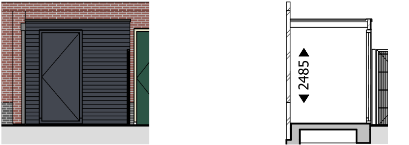
aanzichtdoorsnede
