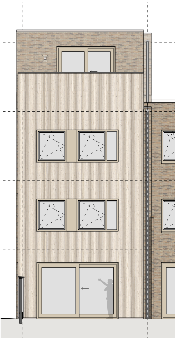
achtergevel bouwnummer 10
