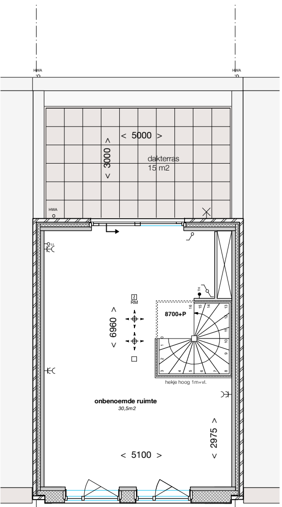
3e verdieping
