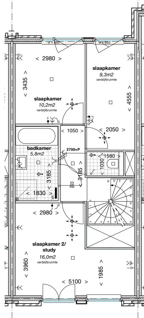
1e verdieping
