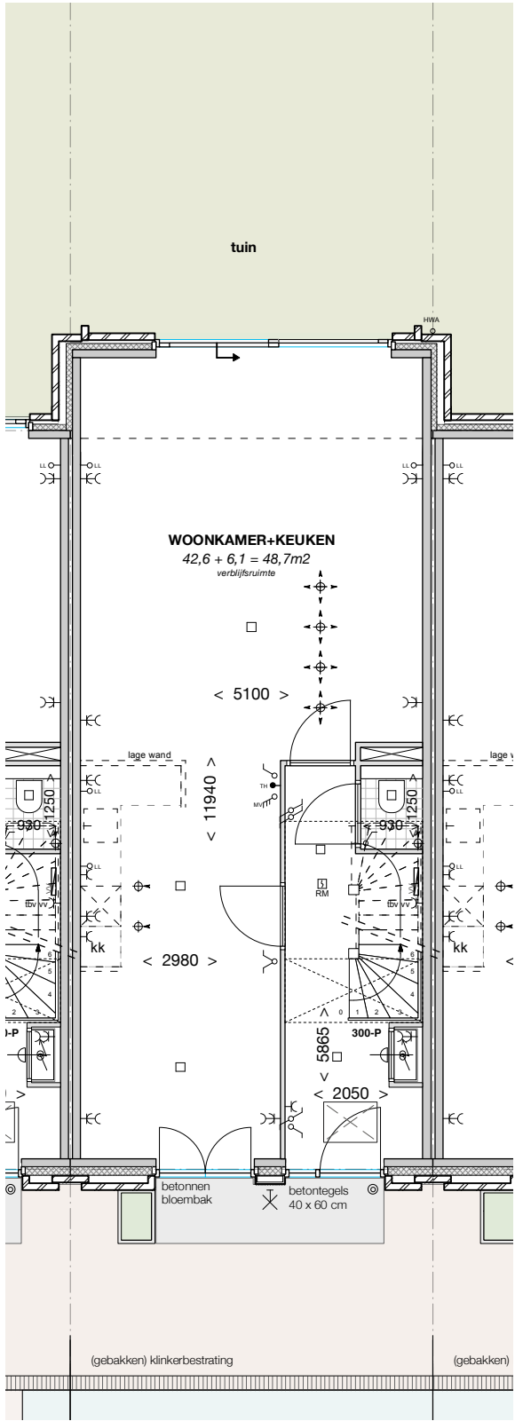
begane grond
