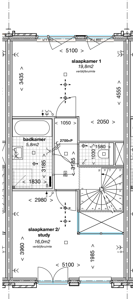
1e verdieping
