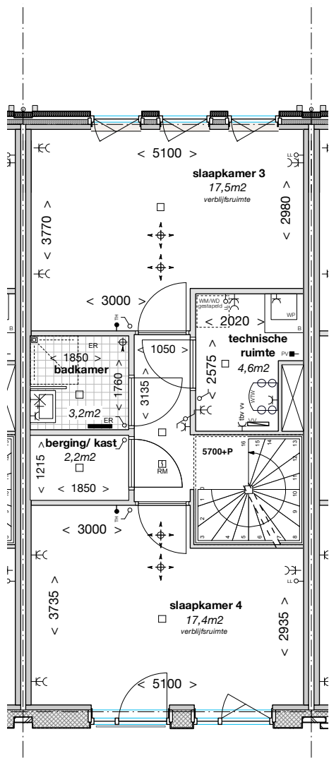
2e verdieping
