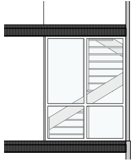
vooraanzicht
